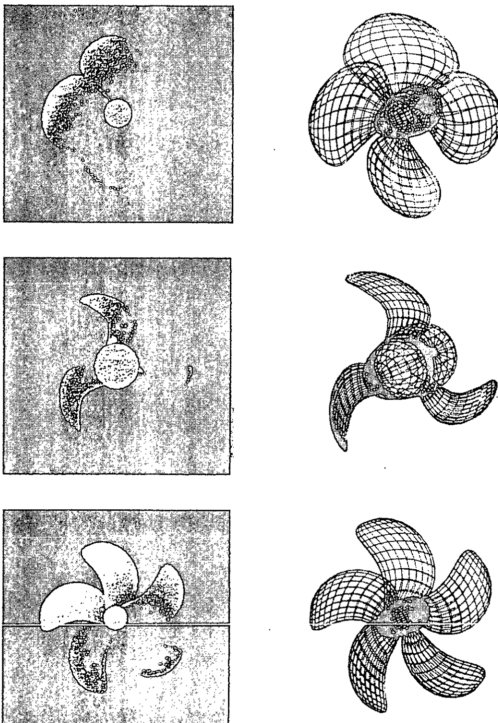
Figura 6: Griglie di calcolo relative ad alcune geometrie di eliche.
