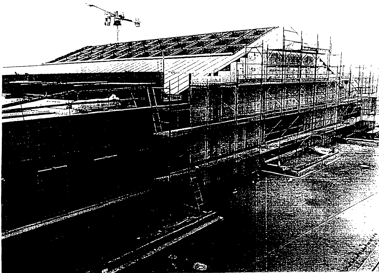
SAVE Aeroporto Marco Polo S.p.a.-Nuova Aerostazione – Zona 1 quota +11,46 chiusura in gasbeton all. 16 ATI: Grandi Lavori Fincosit S.p.a. – ABB Sae S.p.a.
