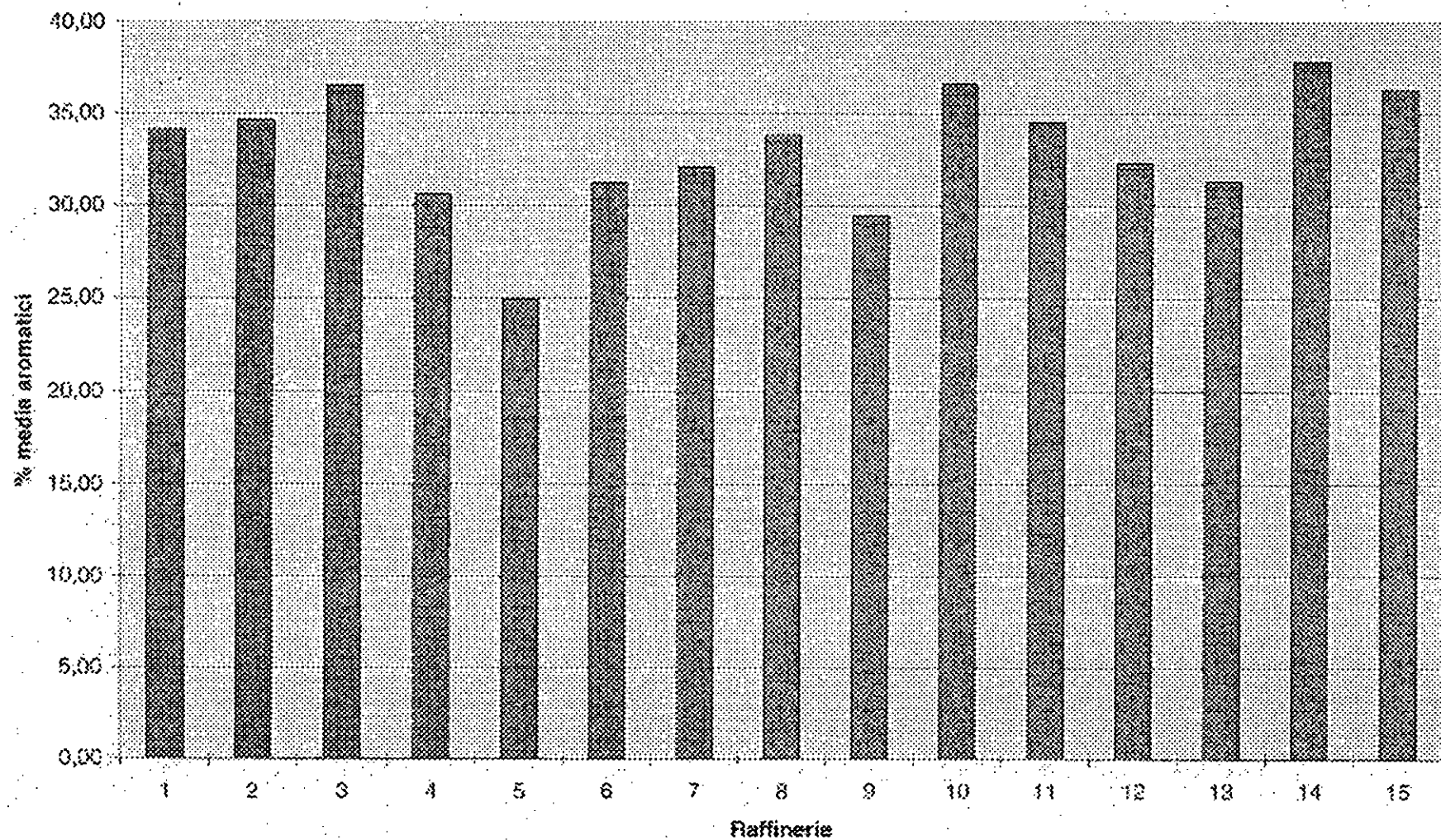
Raffinerie - contenuto % medio di aromatici - produzione anno 1999
