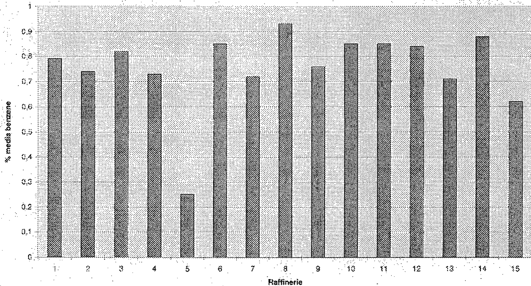
Raffinerie - contenuto % medio di benzene - produzione anno 99 - trim. III o
