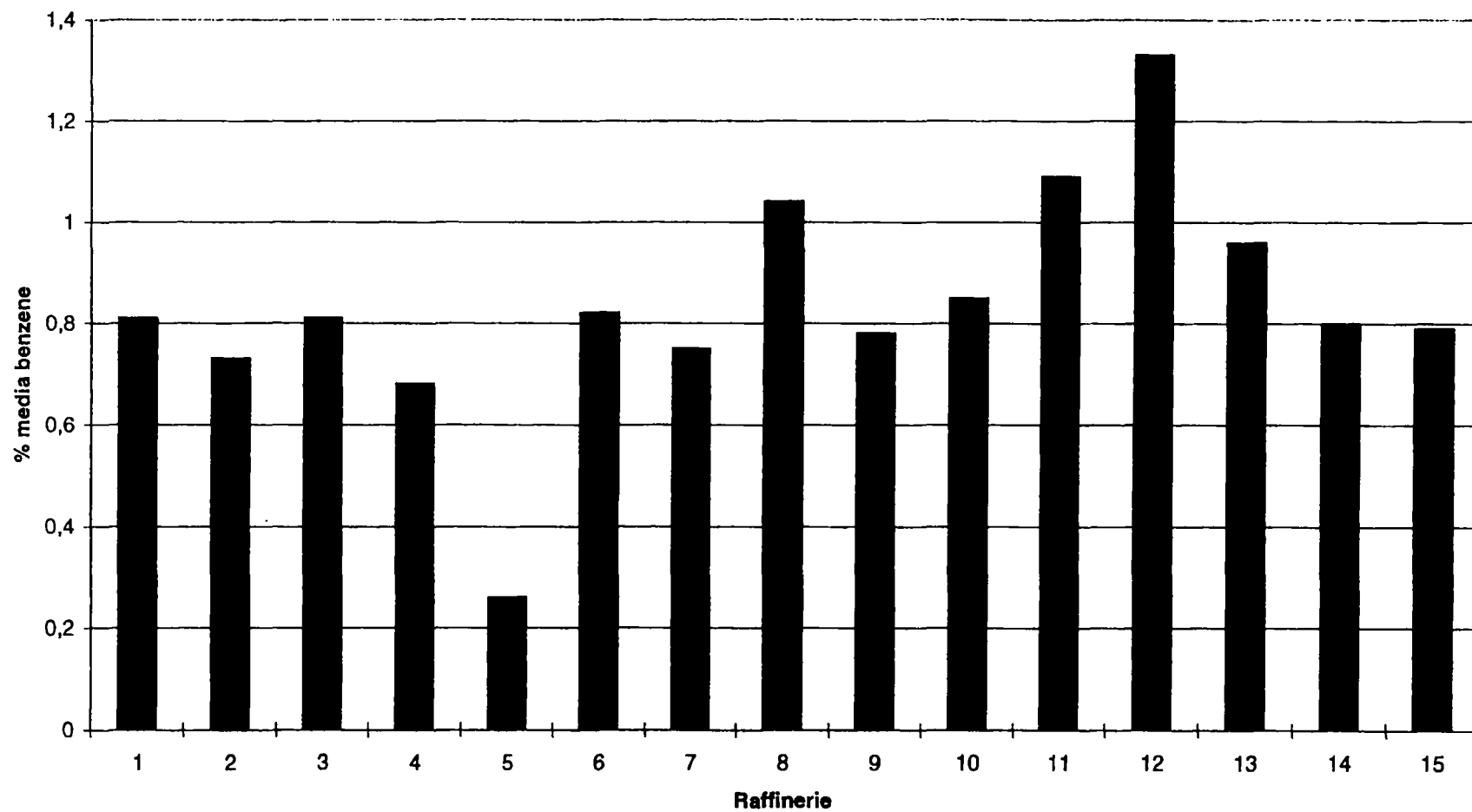
Raffinerie - contenuto % medio di benzene - produzione anno 1998
