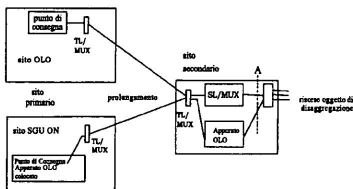
Fig. 3.2: Servizio di prolungamento dell'accesso tra un sito secondario e un sito primario mediante canali numerici
