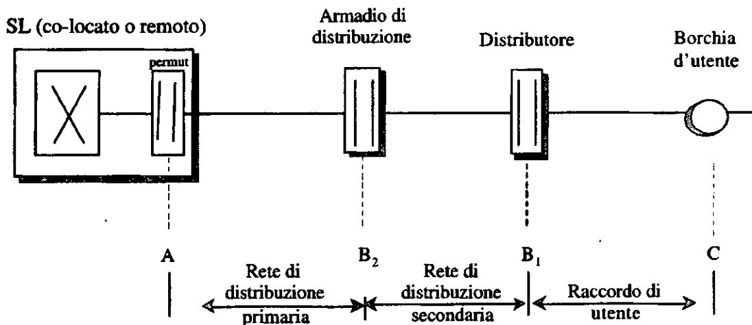
Fig. 1.1. rete di distribuzione in rame
