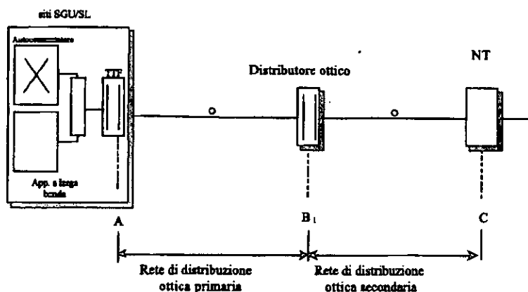
Fig. 1.2. rete di distribuzione in fibra ottica
